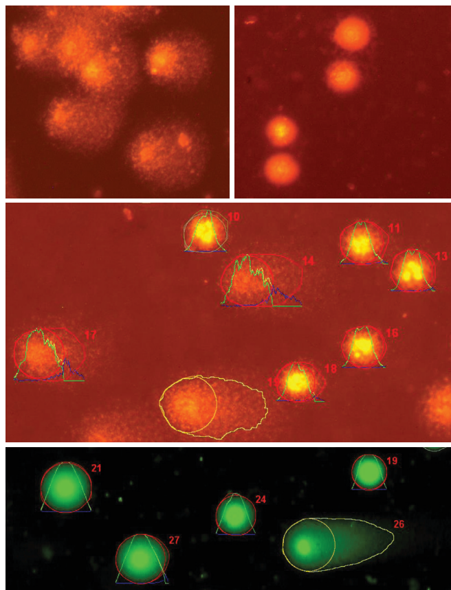
Рис. 1. Микропрепарат ДНК-комет, окрашенный флуоресцентным красителем SYBR Green I (увеличение \times 400 ) (источник: составлено авторами)
