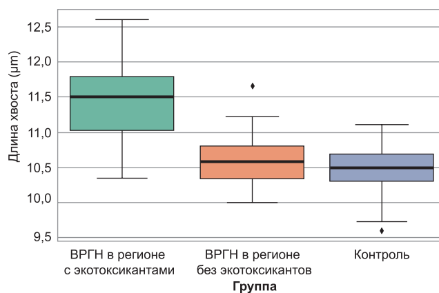
Рис. 2. Распределение и средние значения длины «хвоста» в группах ВРГН в регионе с экотоксикантами, ВРГН в регионе без экотоксикантов и контрольной группе (источник: составлено авторами)
