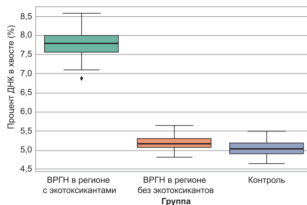
Рис. 3. Распределение и средние значения процента ДНК в хвосте в группах ВРГН в регионе с экотоксикантами, ВРГН в регионе без экотоксикантов и контрольной группе (источник: составлено авторами)
